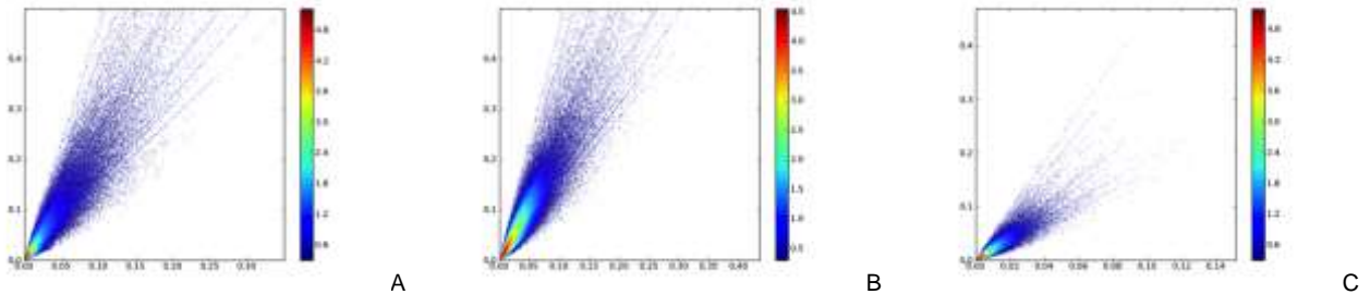
Figure 32-10. SE scatterplots from smoothness parameter 1.0 in X axis and 0.5 in Y axis, A - VIS parameter f_0 , B - VIS parameter f_1 , C - VIS parameter f_2 , Tile h18v04 DOY 145
