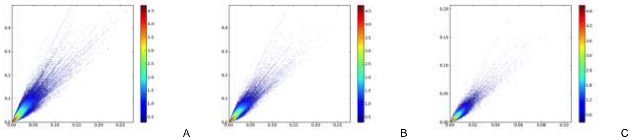
Figure 32-9. Scatterplots of standard error from smoothness parameter 1.0 in X axis and 0.5 in Y axis, A - VIS parameter f_0 , B - VIS parameter f_1 , C - VIS parameter f_2 , Tile h18v04 DoY 001
