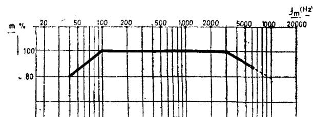
Слика 3 — Зависност на степенот на модулацијата, што предавателот мора да го поднесе во функцијата на фреквенцијата.
