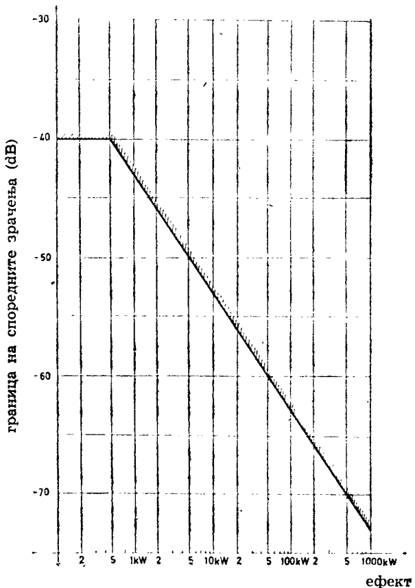
Слика 4 — Средни ефекти на предавателот на која и да било хармонична или споредна фреквенција
