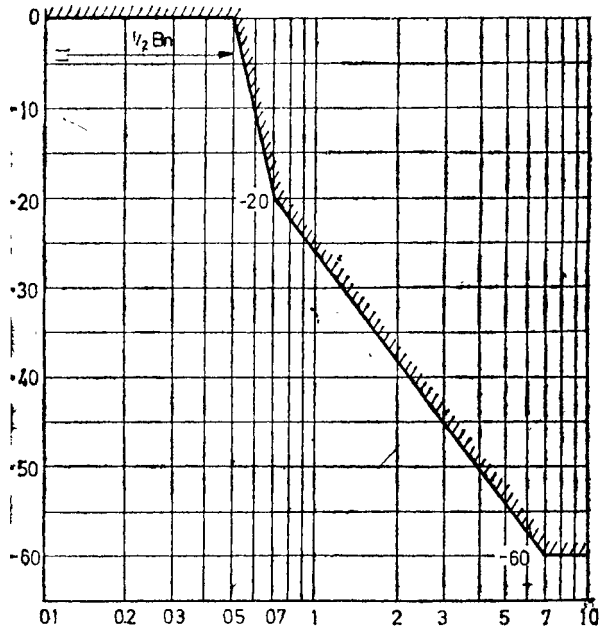
Слика 2 — Дозволените зрачења надвор од потребниот опсег:
