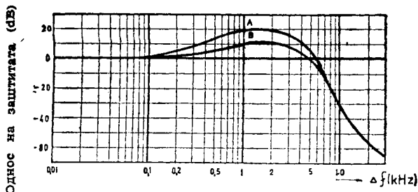
Слика 1 — Заштита во функцијата на фреквентната разлика помеѓу корисниот и попречувачкиот сигнал.
