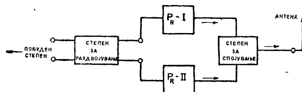
Слика 5 — Удвоени радиодифузни предаватели
